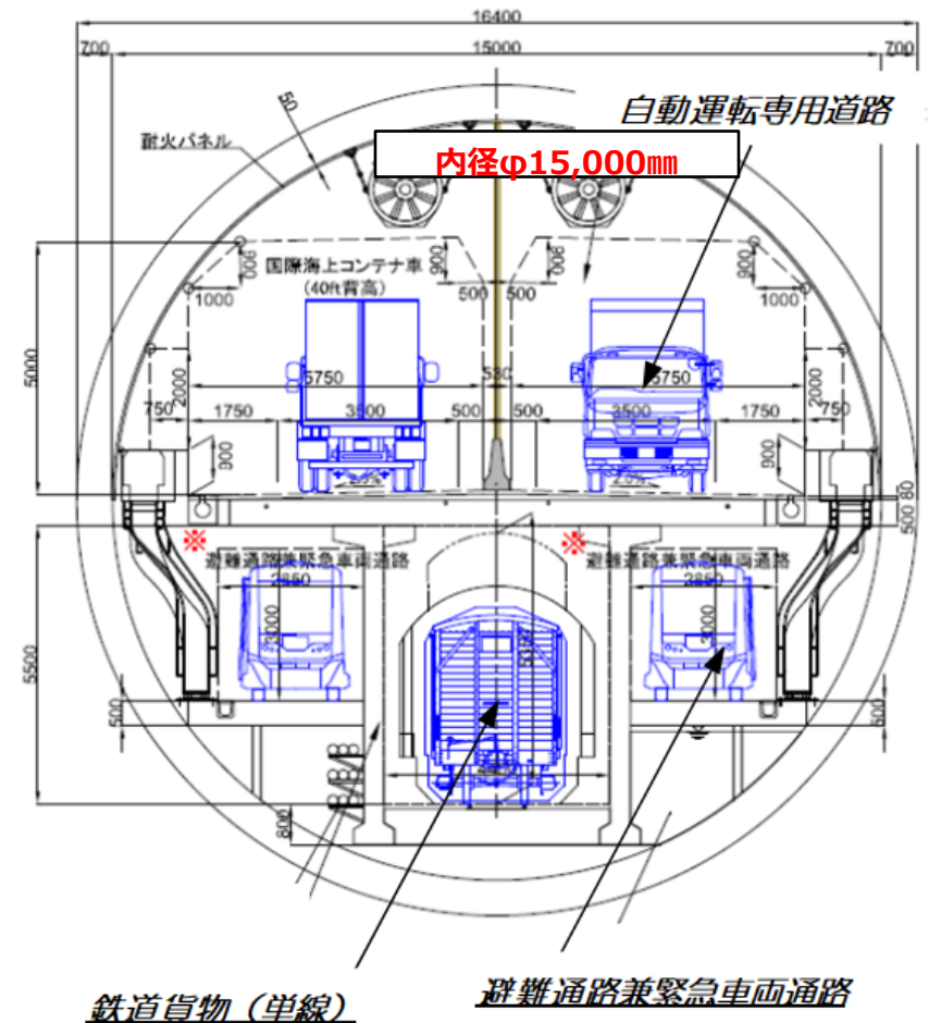
トンネル断面(内径φ15m)
