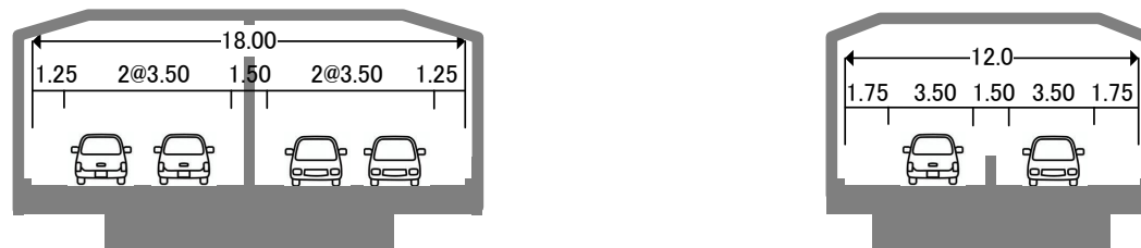
【高架構造】
